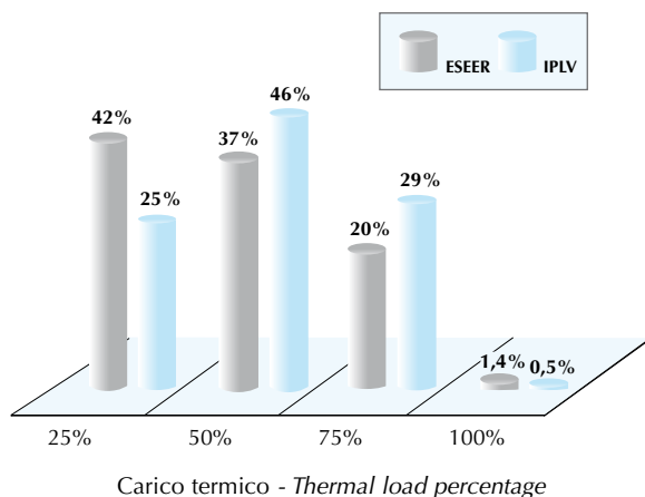
Percentuali di tempo di funzionamento secondo ESEER e IPLV ESEER and IPLV operating time percentages
