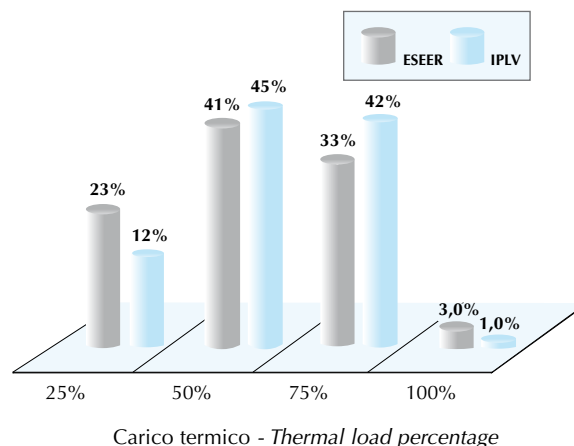
Pesi energetici secondo ESEER e IPLV ESEER and IPLV energy weights
